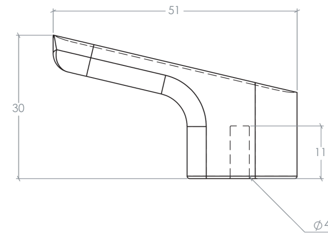
Pull Knob
